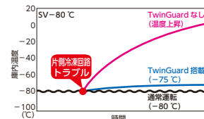
■コンプレッサー片側運転温度推移イメージ
