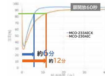
■器内湿度復帰時間イメージ
