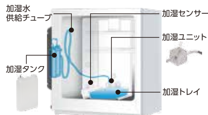
■アクティブ加湿システムイメージ
